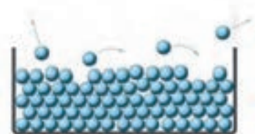
شکل ۴-۳۳ در حین تبخیر سطحی، مولکول‌های پرانرژی‌تر از سطح مایع می‌گریزند.
